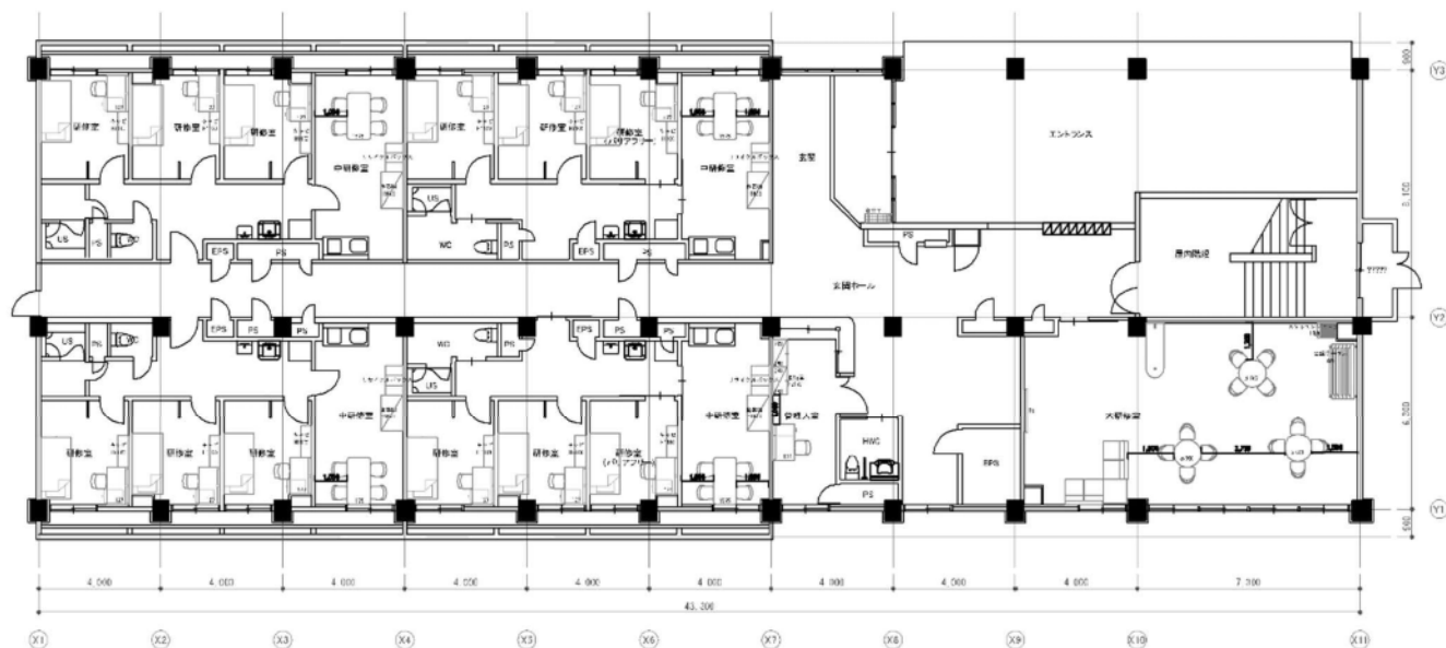
1階平面図
