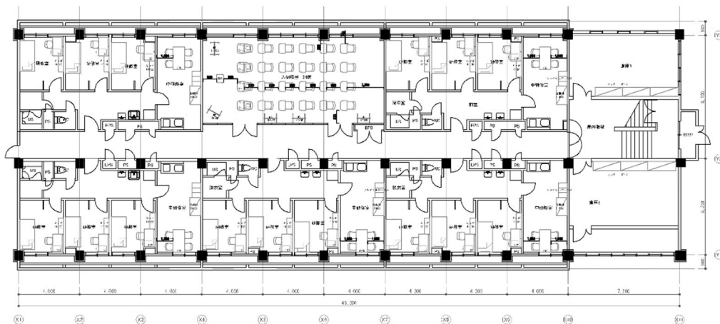
2・3階平面図
